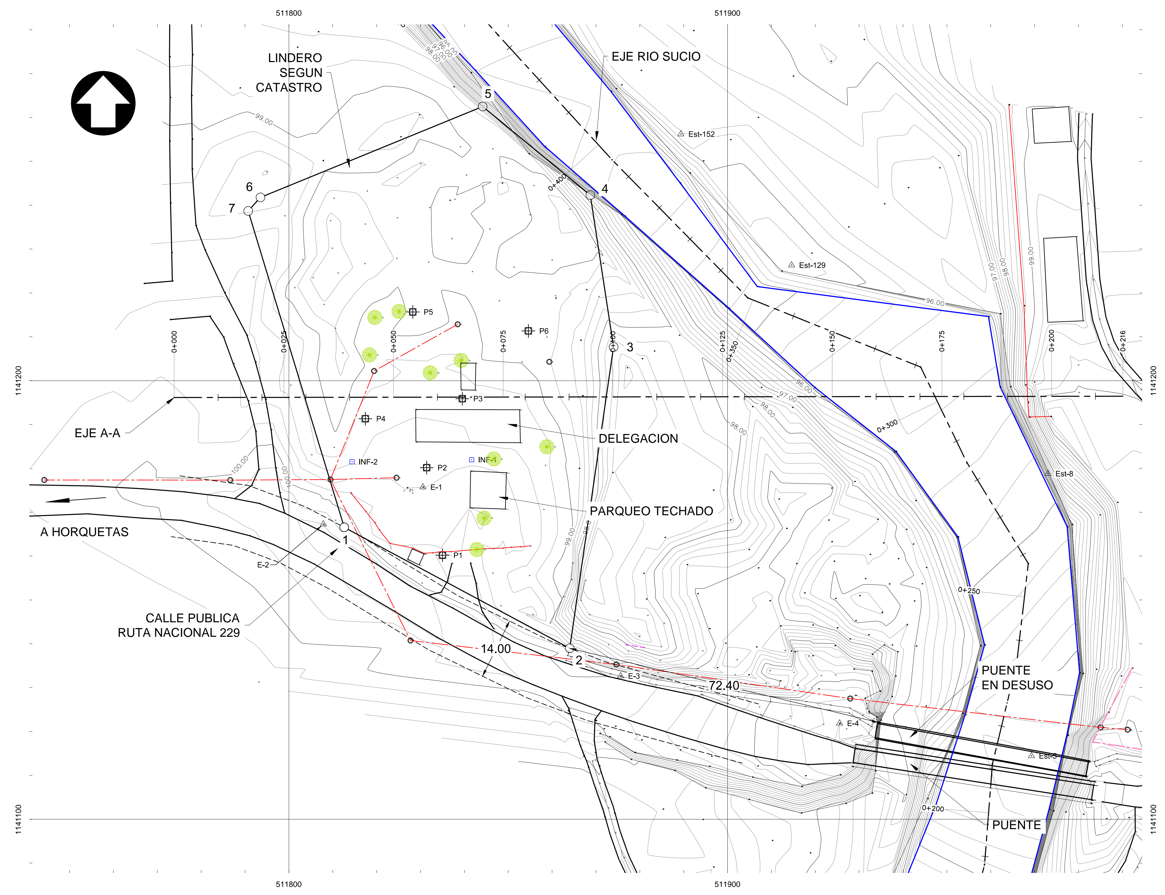
AREA DELEGACION POLICIAL DE RIO FRIO ESCALA HORIZONTAL 1 : 500
