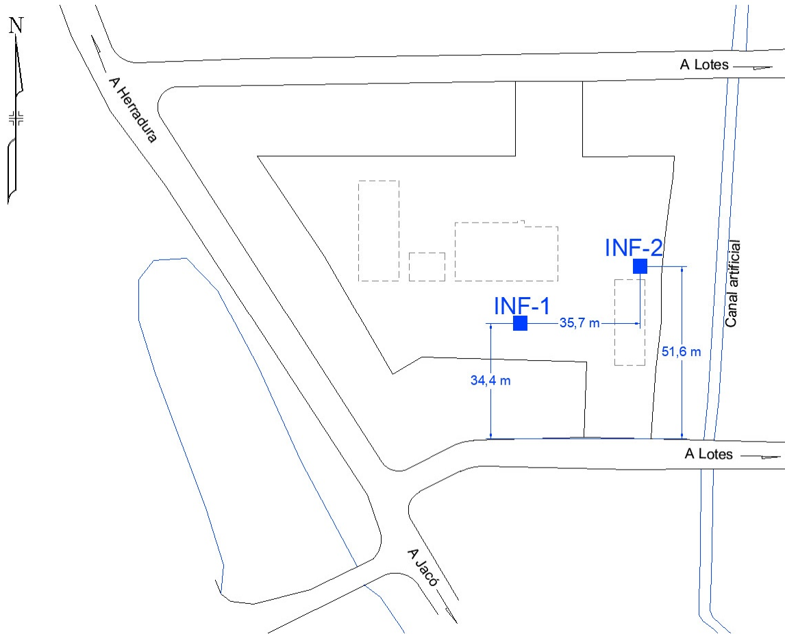
Figura. Diagrama de distribución de prueba de infiltración. Nota: Las medidas son aproximadas.
