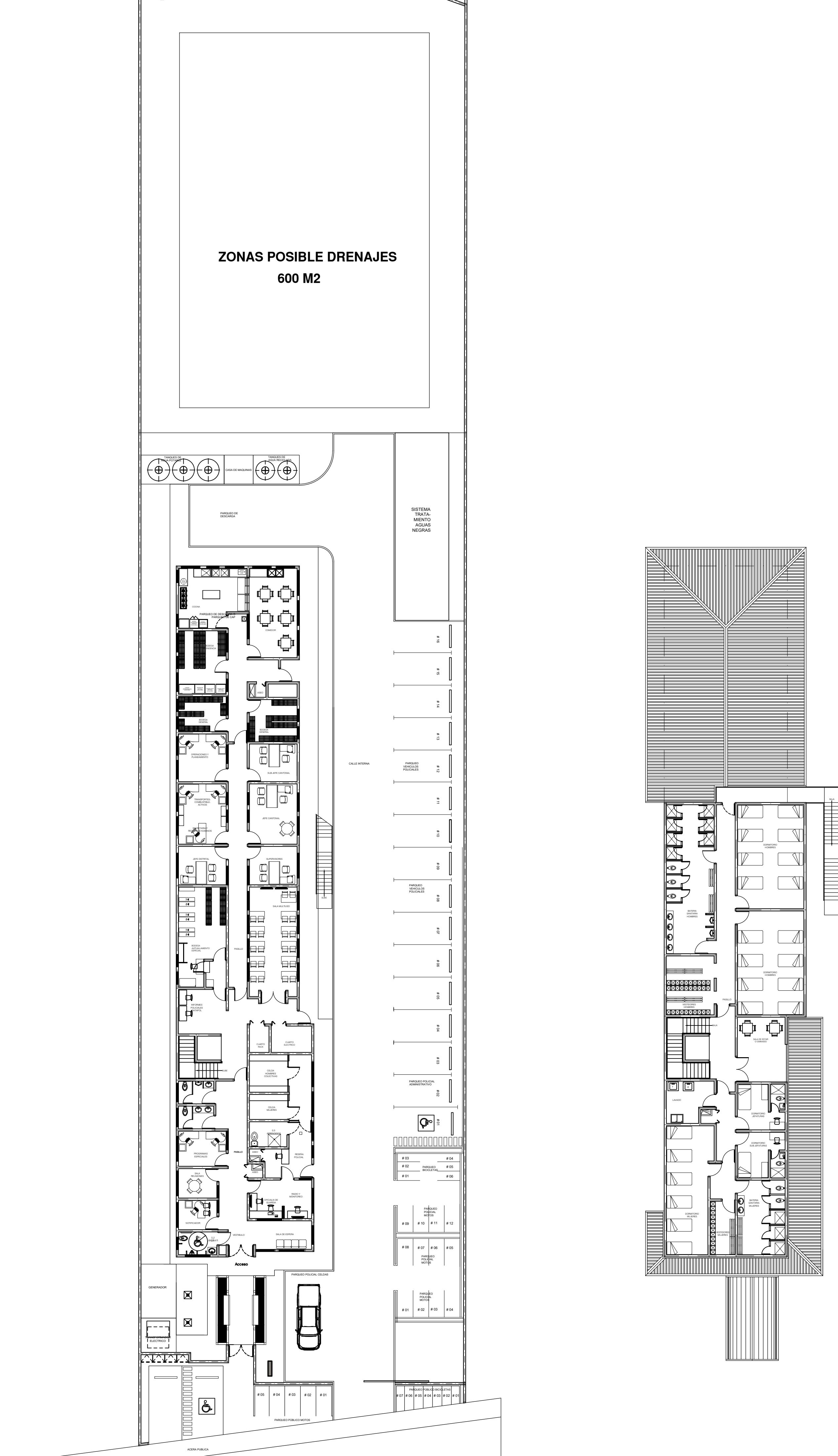
Planta Distribución Arquitectónica Modelo Delegación Cantonal Siquirres SEGUNDO NIVEL Esc. 1:200 AREA TOTAL 385 M 2
